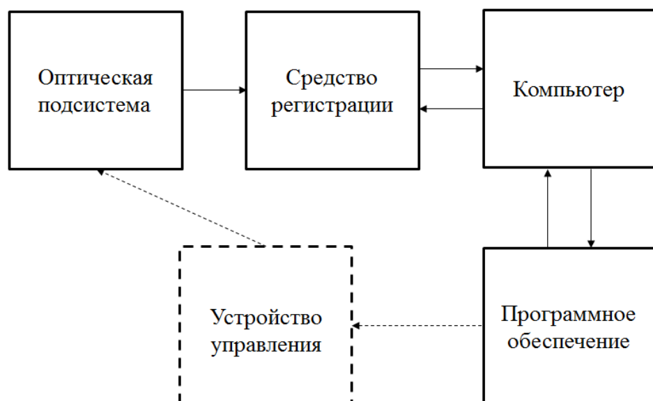
Рисунок 5 – Общая схема системы неразрушающего контроля.
